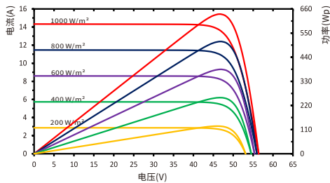
不同辐照度下, I-V 曲线图
